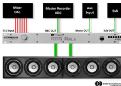
Kopplingschema
